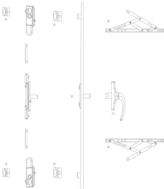
WK100 外开平窗五金配置表
